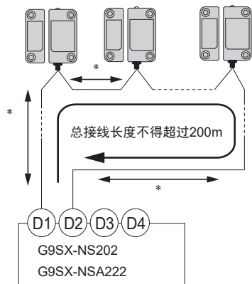
* 产品间的接线长度不得超过100m。
