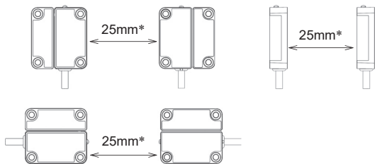
* 与D40Z相邻时：50mm
